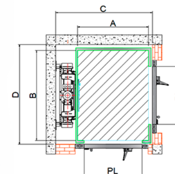
Entradas Adjacentes
