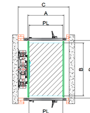
Entradas Opostas
